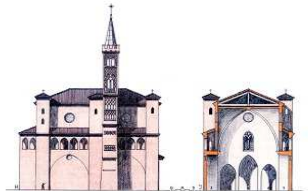
H. Alzado representativo. J. Sección transversal oriental. 3. Capilla San Gil. 4. Capilla Nra. Señora. 5. Capilla del Santísimo. 6. Capilla San Juan Evangelista. 7. Capilla Sta. Fe. 10. Galerías
