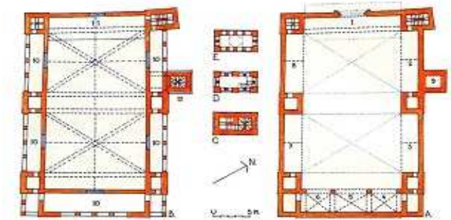
Planta Baja: 1. Acceso (Cofre Órgano). 2. Capilla de Santa Ana. 3. Capilla San Gil. 4. Capilla Nra. Señora. 5. Capilla del Santísimo. 6. Capilla San Juan Bautista. 7. Capilla Santo Fe. 8. Capilla San Cristóbal. 9. Arranque del Campanario. 10. Galerías. 11. Coro. Campanario. 12. Primer cuerpo. C.: Cuerpo 2º. D.: Cuerpo 3º. E.: Piso Superior.
